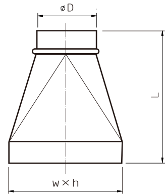
前視圖
